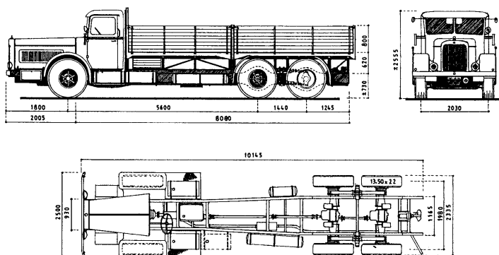
HENSCHEL 36 W 3
